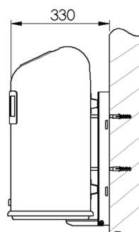
Wandbefestigung
