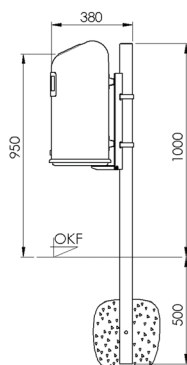
Pfostenbefestigung
